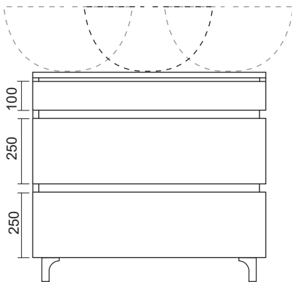
Art. FRTOP80 Top in legno e sifone salvaspazio
